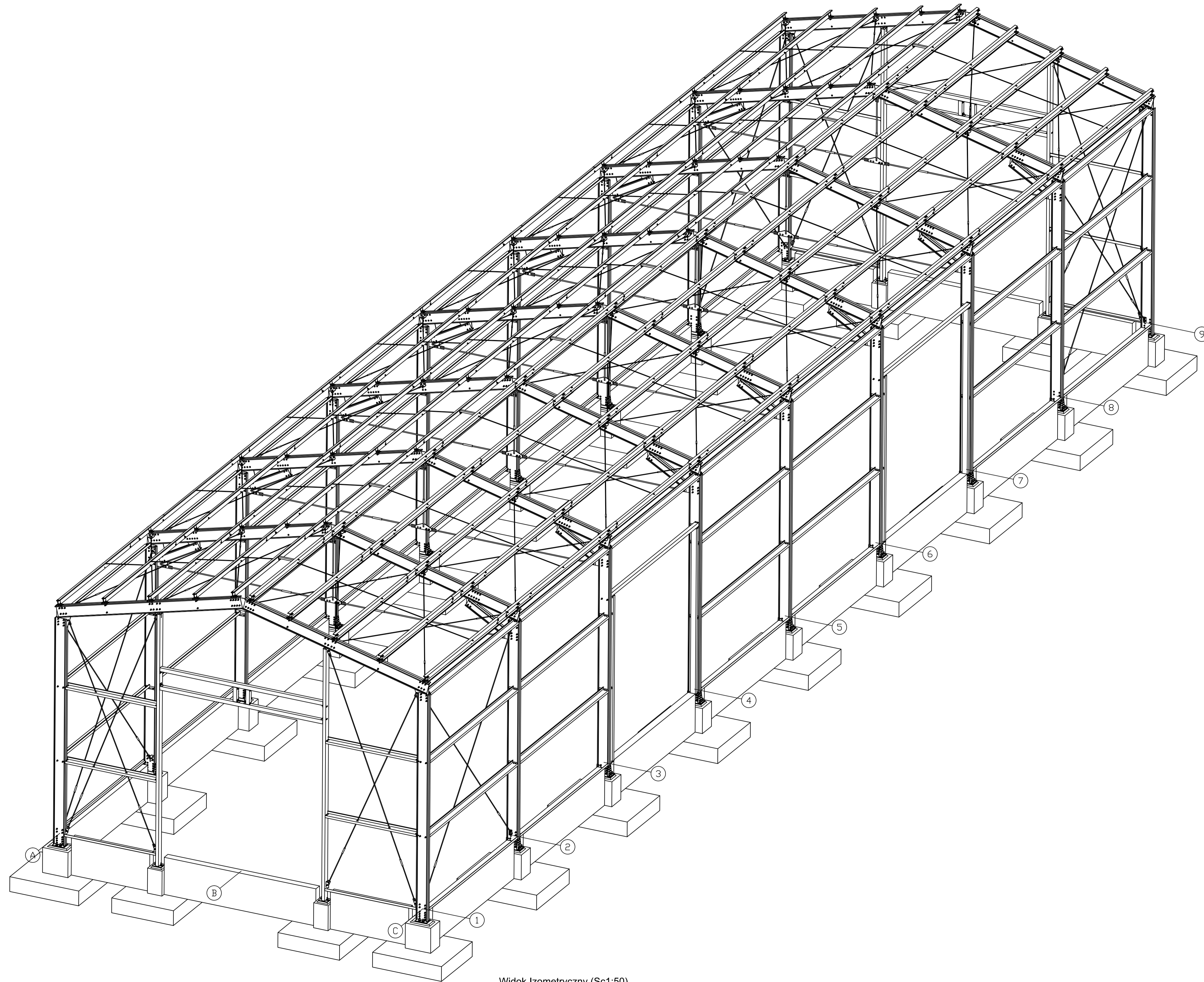
Widok Izometryczny (Sc1:50)
